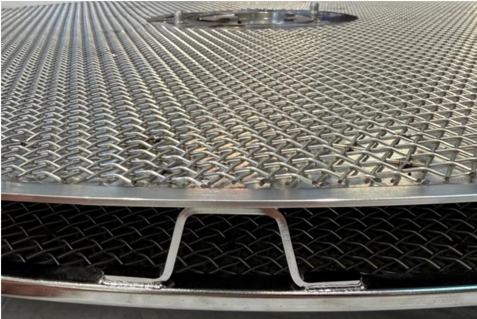
Filterplatten für SeitzSchenk-ZHF-Druckplattenfilter (Bild: Chemap).
