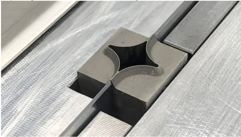
Bandstahlwerkzeug zum Querstanzen von Aufschnittverpackungen (Bild: Marbach).
