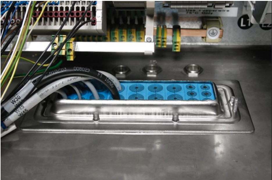
Flexible Kabel- und Leitungsabdichtung im Rahmen aus Edelstahl (Bild: Roxtec).
